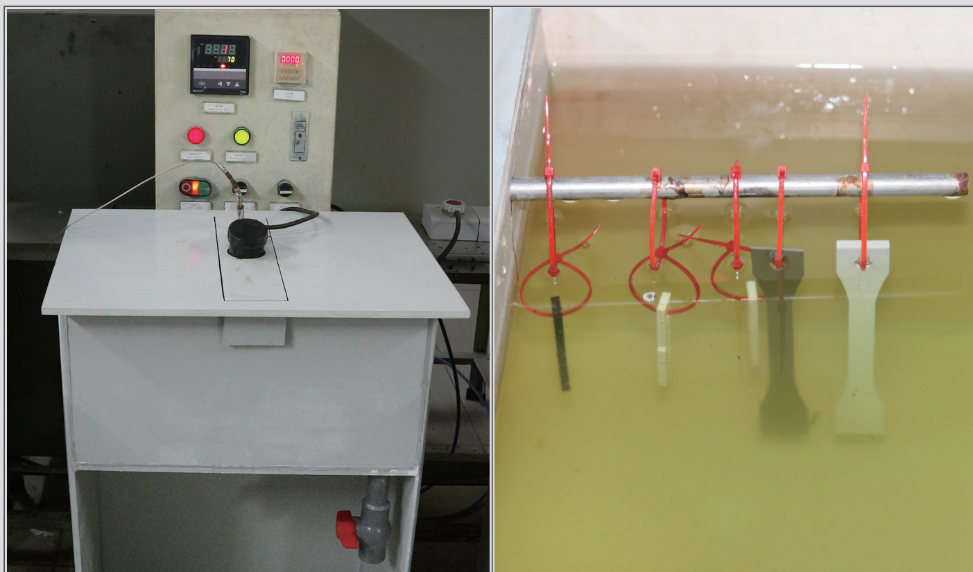
Bain d'essai de la résistance à la corrosion au chlore réalisé dans notre laboratoire
