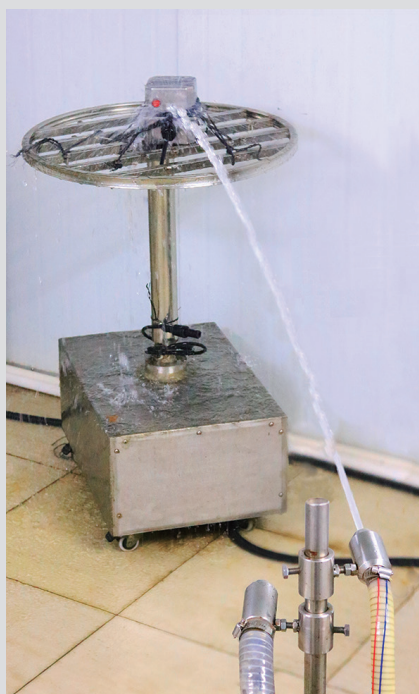
IPx5 test
