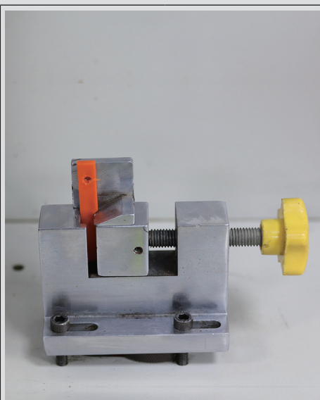
Eprouvette avant essai Charpy
